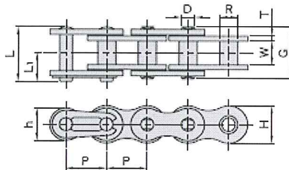
図1 形状
